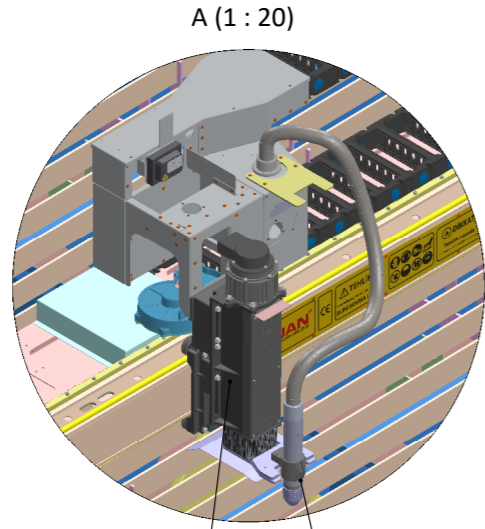
THC Ünitesi THC Unit Plazma Torçu Plasma Torch
